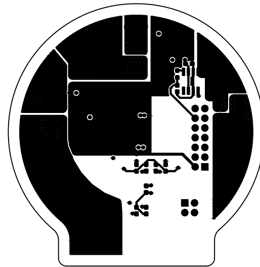
Проводящий рисунок 21
