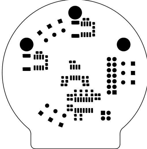
Защитная паяльная маска рисунок 12
