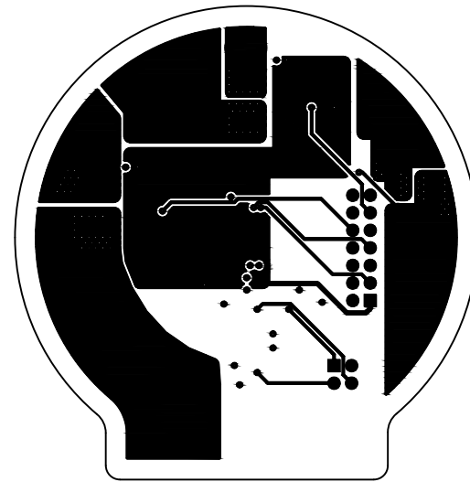
Проводящий рисунок 12
