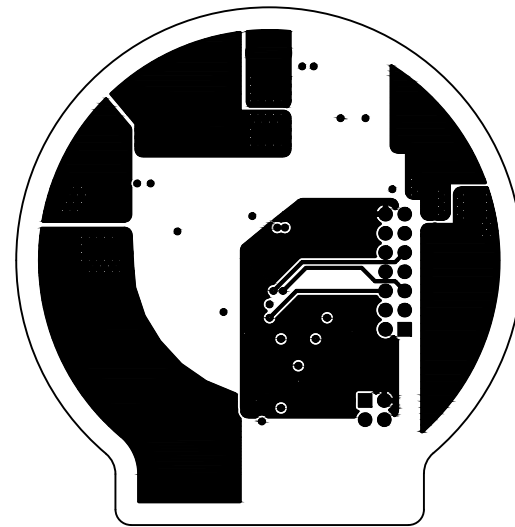
Проводящий рисунок 22
