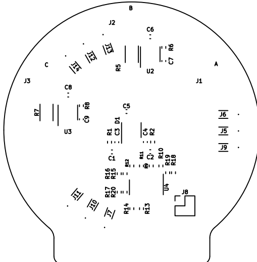
Шелкография рисунок 12
